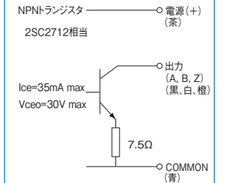
オープンコレクタ出力
