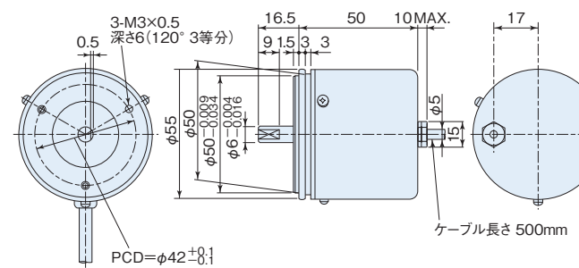
MESW-45(オプション:防滴タイプ)
