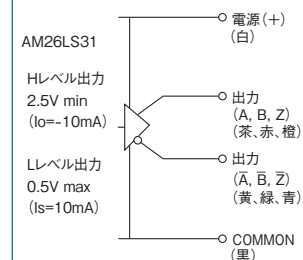
差動ドライバ出力
