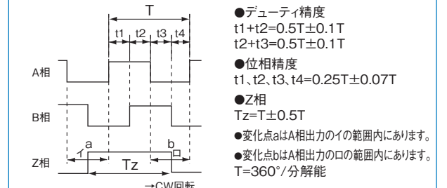
電圧出力・オープンコレクタ出力
