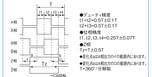
差動ドライバ出力
