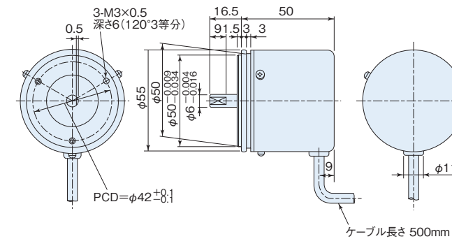
MES-45(標準タイプ)
